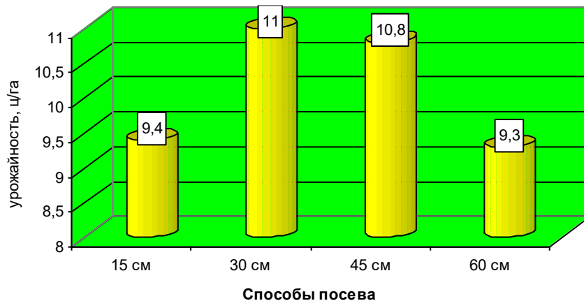
Влияние способов посева на урожайность нута
