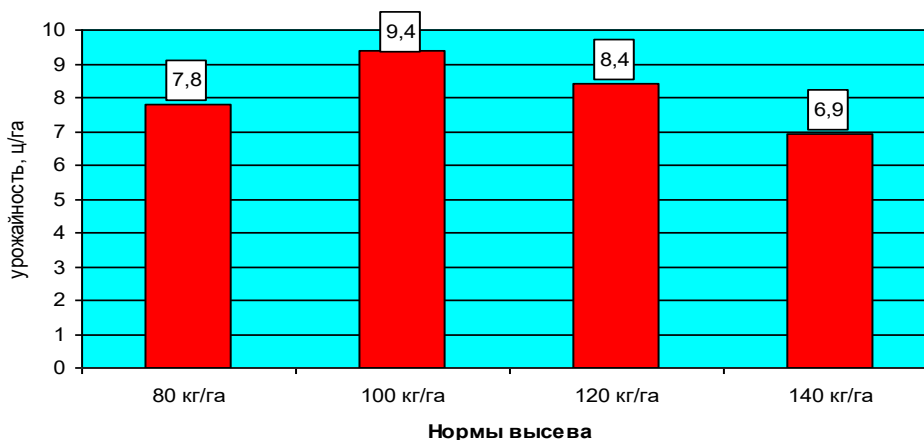
Влияние норм высева на урожайность нута
