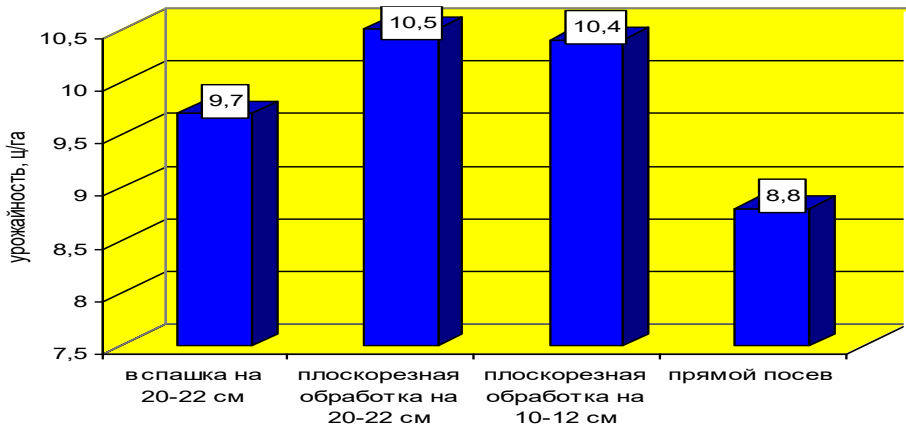
Влияние приемов обработки почвы на урожайность нута
